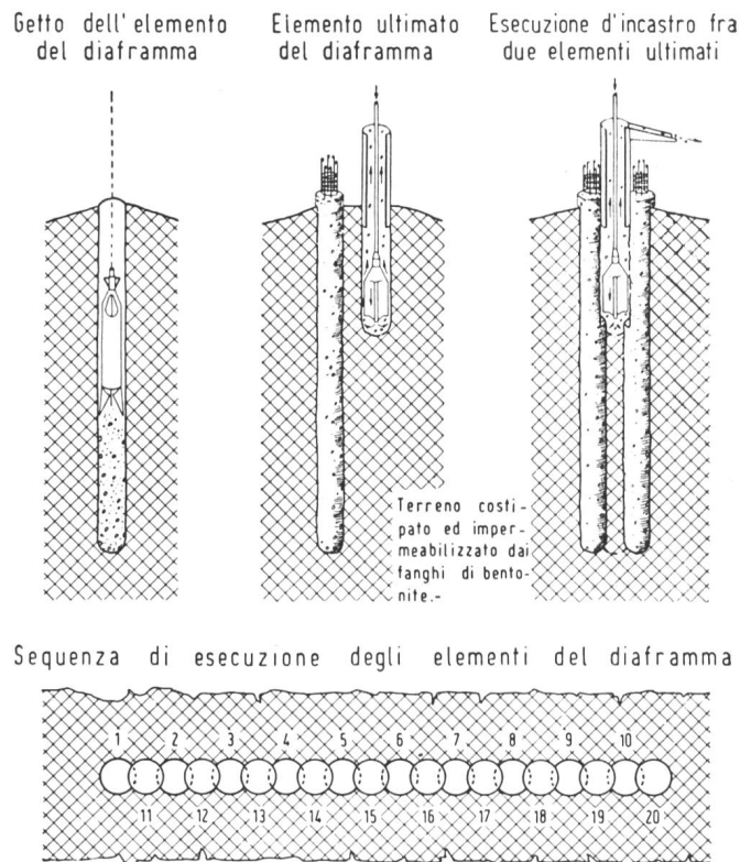
Abb. 28 Staudamm Fedaia, Ausführungsschema für das Dichtungsdiaphragma
