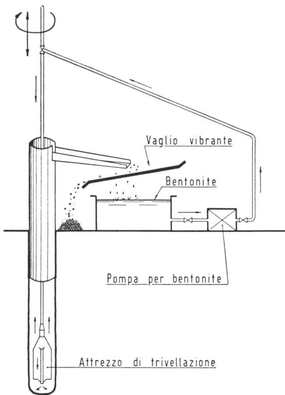
Abb. 28 Staudamm Fedaia, Ausführungsschema für das Dichtungsdiaphragma
