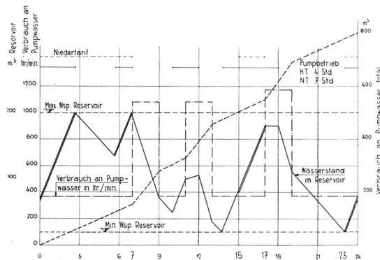
Bild 3 Das theoretische Tages-Diagramm — für einen ungünstigen Wintertag — gibt den Wasserstand im Reservoir, den Pumpwasserverbrauch und die Pumpenbetriebsstunden, wobei diese nach Möglichkeit auf die Zeit des Niedertarifes verlegt werden. Das Diagramm basiert auf folgenden Annahmen:
