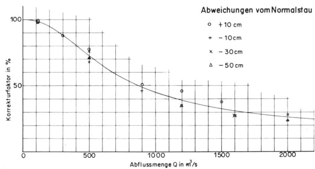
Bild 3 Korrekturfaktor in Funktion der Abflussmenge für die Station 1
