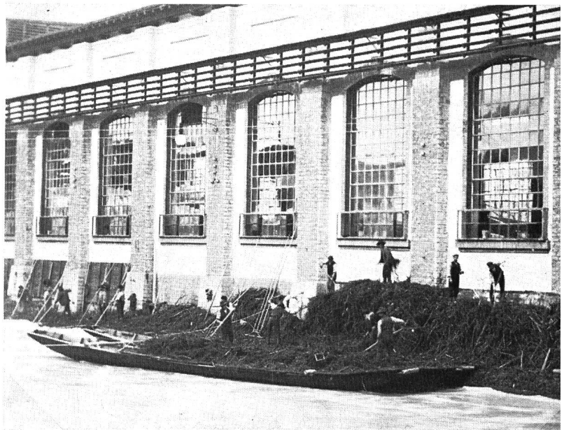
Bild 1 Geschwemmselantrieb des Hochwassers 1910 beim Kraftwerk Rheinfelden
