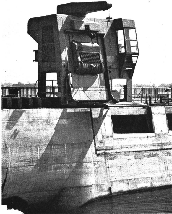
KW. Strassburg Rechenreinigungsmaschine mit Turmdrehkran
