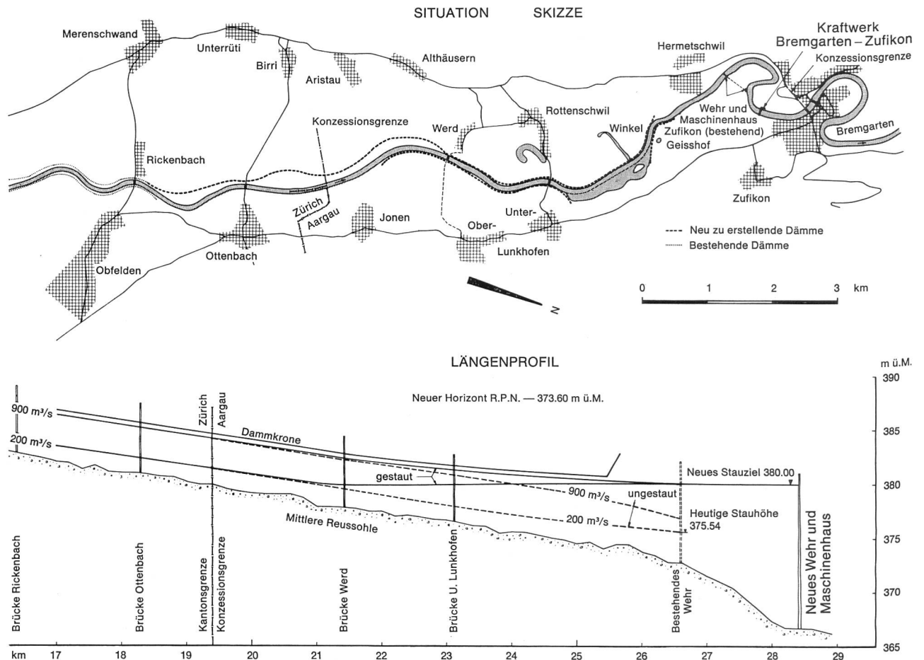
Bild 2 Reusskraftwerk Bremgarten-Zufikon, Lageplan und Längenprofil.
