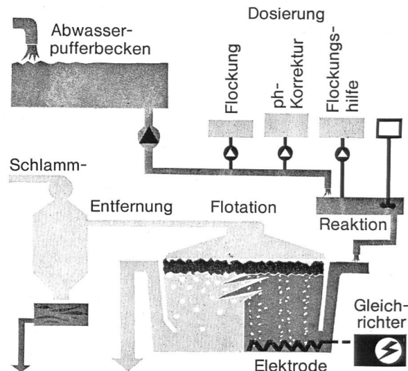
Bild 3 Elektroflotation-Einrichtung.
