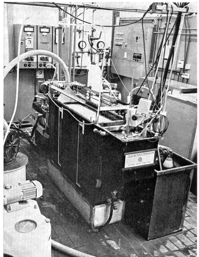
Bild 13 Gesamtübersicht einer Pilotanlage.
