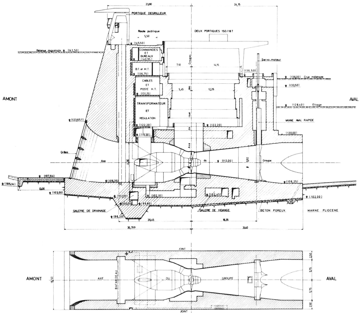
Bild 10. Rhonestufe le Péage-de-Roussillon. Vertikalschnitt durch die Zentrale (oben) und Horizontalschnitt durch eine Rohrturbine (unten), Masstab 1:500. Figure 10. Aménagement du Péage-de-Roussillon. Coupe transversale à travers l'usine hydro-électrique (en haut) et plan-coupe d'un groupe (en bas), à l'échelle 1:500.
