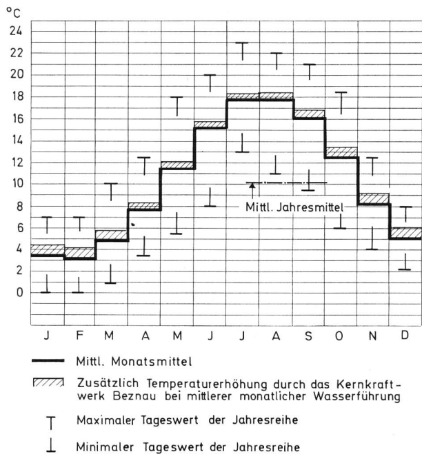
Bild 8. Monatsmittel und Tagesextrema 1950 bis 1969 der natürlichen Aarewassertemperaturen bei der Beznau. Schraffiert die Monatsmittel der Temperaturerhöhungen in der Aare infolge der Abwärme des Kernkraftwerks Beznau bei Vollast, nach voller Durchmischung und bei einer Wasserführung der Aare entsprechend dem langjährigen Monatsmittel.
