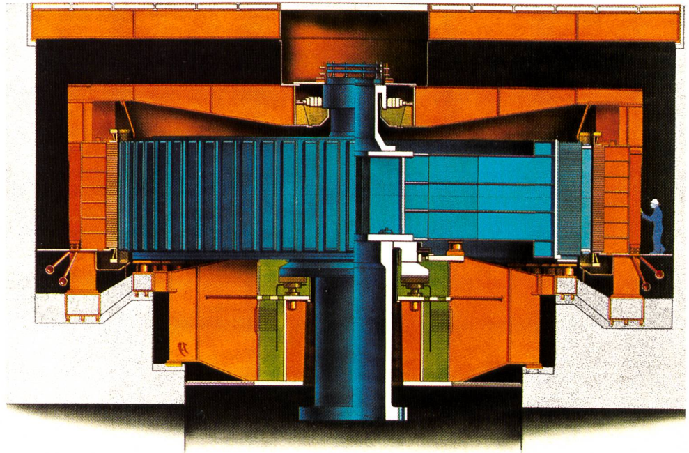
Bild 10. Kraftwerk Itaipu/Brasilien-Paraguay. Schnitt durch den Generator.
