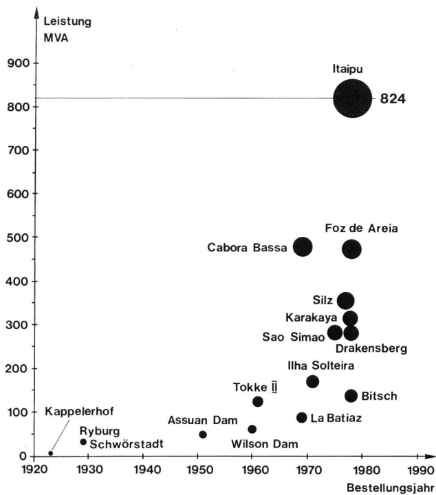
Bild 12. Steigerung der Einheitenleistung von Wasserkraftgeneratoren in den letzten 50 Jahren.
