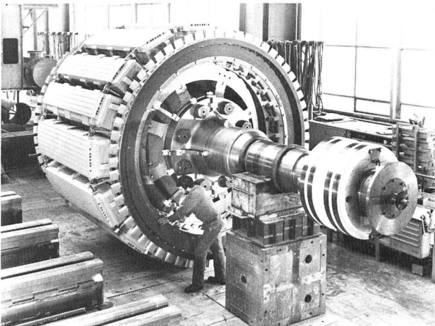
Bild 5. Kraftwerkgruppe Malta. Motor-Generator für das Krafthaus Oberstufe. Polrad bei der Werkmontage.
