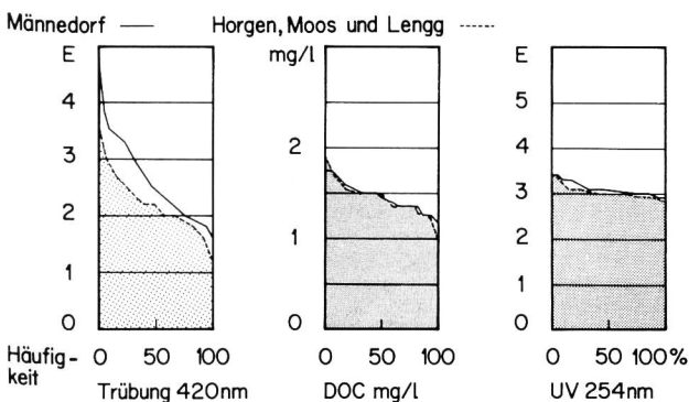
Bild 21. Die Häufigkeitsverteilung der Werte Trübung, DOC und UV 254 nm im Rohwasser der Werke Mändedorf, Horgen, Moos-Zürich und Leng-Zürich.
