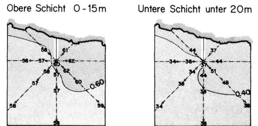
Bild 23. Trübungsmessungen vom 1. September 1978 an der Fassungsstelle Mändedorf; Extinktion bei 420 nm. Massstab 1:60 000.
