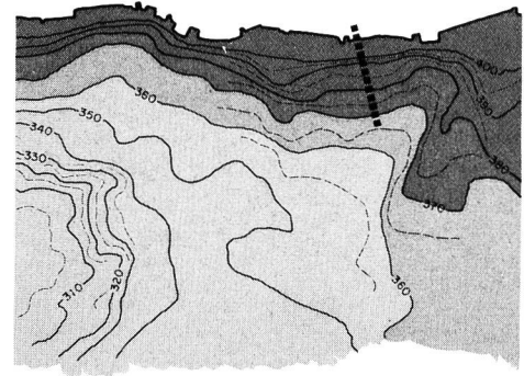
Bild 22. Topographie des Seegrundes an der Fassungsstelle Mändedorf. Massstab 1:35 000.
