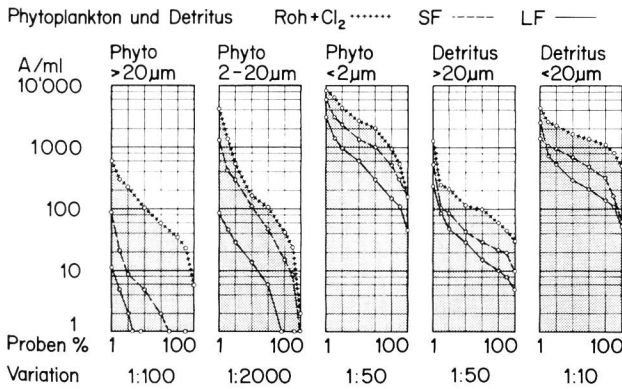
Bild 19. Die Häufigkeits-Dauerkurven von Phytoplankton und Detritus im Rohwasser des Seewasserwerkes Moos; 1974/1975.
