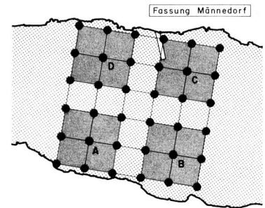
Bild 24. Synoptische Messungen am Zürichsee im Planquadrat Mändedorf — Stäfa — Wädenswil vom 29. bis 31. August 1978 (57 Stunden). Massstab 1:90 000.
