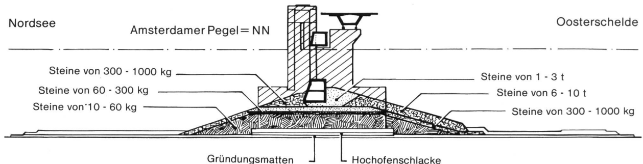
Bild 9. Aufbau der Wehrrundung und Umschüttung.
