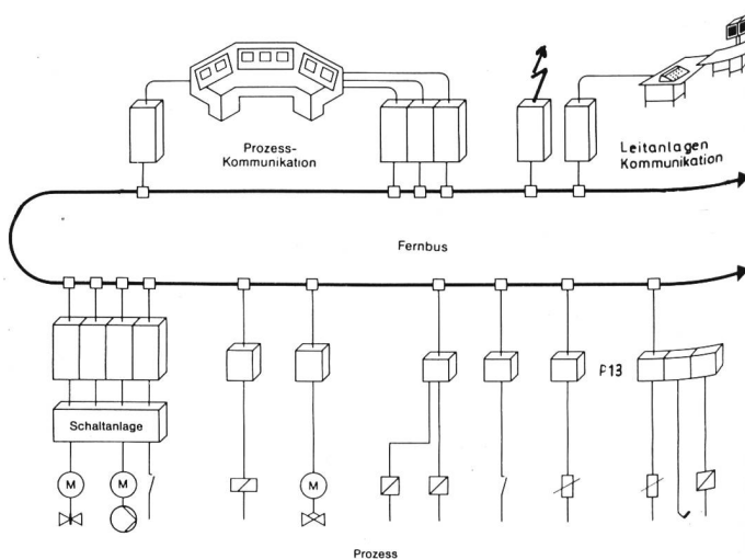
Bild 1. Konfiguration des Kraftwerk-Leitsystems «Procontrol P».
