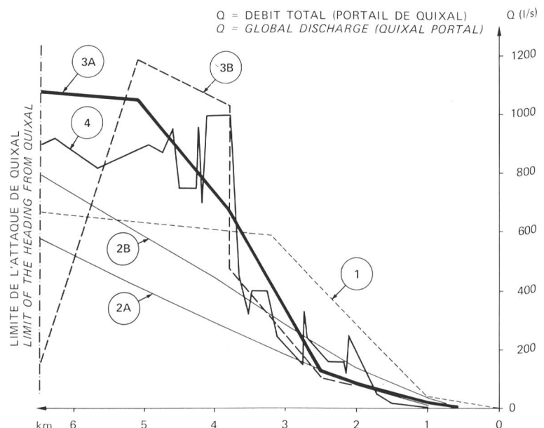
Figure 3. Galerie d'aménée Agua Blanca – Quixal, Débits cumulés en fonction de l'avancement (prévisions et observations).
