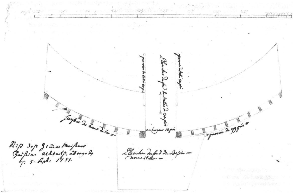
Bild 2. Grundriss von 1751 der Bogenstaumauer Joux-Verte oberhalb Roche/VD.
