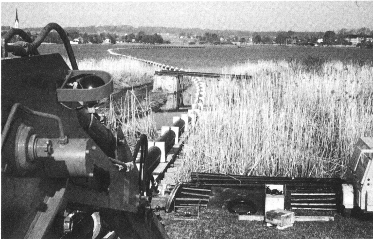
Bild 3, links. PE-Leitung in der Verlegetrasse. Bild 5, rechts. Anschlussschweissung eines schwimmenden Teilstranges im Traunsee.
