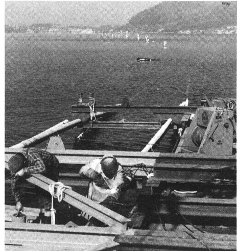
Bild 3, links. PE-Leitung in der Verlegetrasse. Bild 5, rechts. Anschlussschweissung eines schwimmenden Teilstranges im Traunsee.
