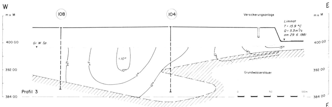
Bild 12b. Temperaturverhältnisse im Grundwasser am 29. Juni 1981 ohne Rückversickerung.
