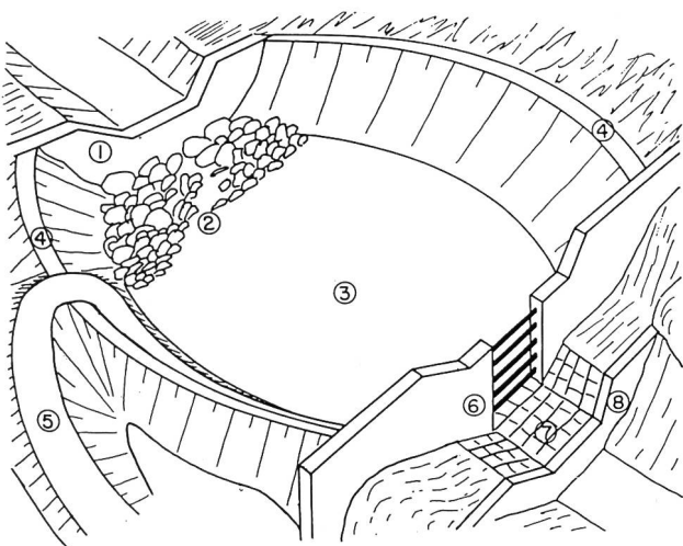
Bild 1. Geschiebeablagerungsplatz mit seinen Teilen: 1 Einlaufbauwerk, 2 Kolkabsicherung, 3 Ablagerungsplatz, 4 Umfassungsdämme, 5 Zufahrtstrasse (Leerung), 6 Rückhaltebauwerk, 7 Kolkabsicherung, 8 Gegensperrung.
