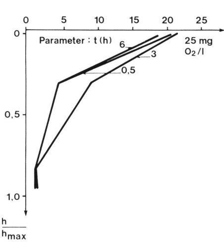
Bild 4. O 2 -Profile nach verschiedenen Filterlaufzeiten.
