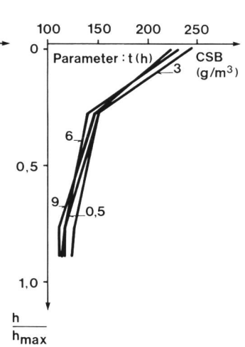
Bild 5. CSB-Profile nach verschiedenen Filterlaufzeiten.
