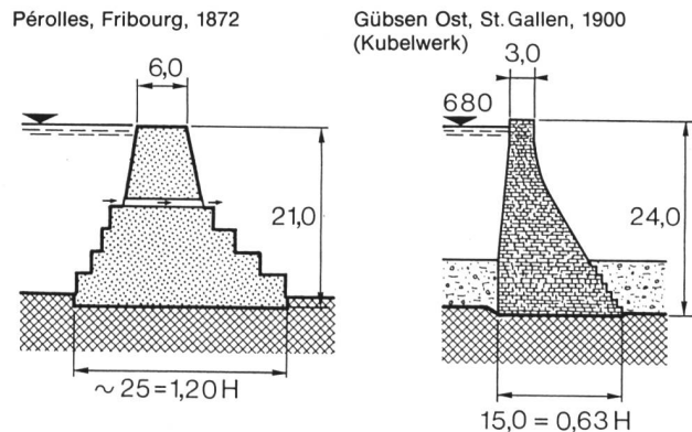
Bild 11. Querschnitte zweier früher schweizerischer Gewichtsstau-mauern; linke über-, rechte unterdimensioniert und 1986 verstärkt.
