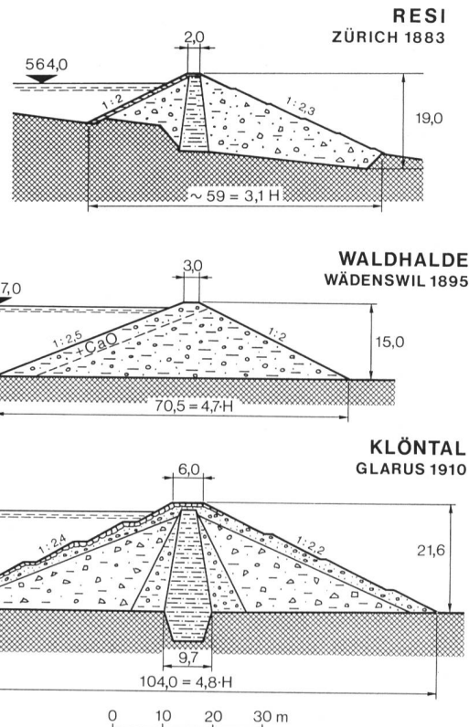
Bild 12. Querschnitte dreier früherer Erddämme in der Schweiz.
