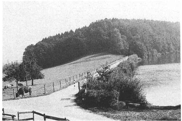
Bild 2. Der Norddam des Gübsensees, von Westen her gesehen. Damit seine Standfestigkeit und Dichtigkeit auch weiterhin gewährleistet ist, mussten auf dem Dam gewachsene grössere Bäume entfernt werden. In der Mitte des Dammes (unter dem Weg) wurde eine 2,5 m tiefe Beton-trennwand eingefügt, um den Dam abzudichten.
