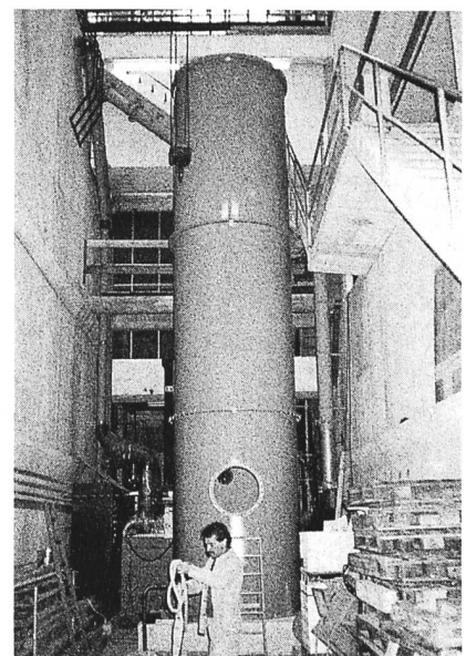
Figure 4. Tank à niveau constant simulant un bassin de retenue pour l'étude de la vanne équipant l'entrée de la galerie en charge. Hauteur du tank 8,1 m; diamètre 1,8 m.
