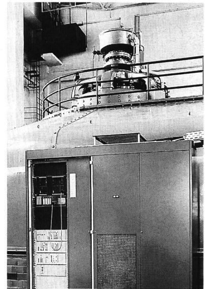
Wasserkraftwerk Rekingen. Statische Erregung mit digitalem Spannungsregler.
