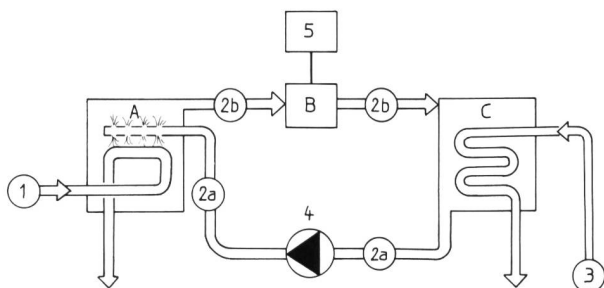
Bild 5. Schema der Wärmeenergienutzung im geschlossenen Kreislauf (Zeichnung: Cyrrill Engel ). A Verdampfer, B Niederdruckdampfturbine, C Kondensator, 1 Kreislauf des warmen Oberflächenwassers, 2 Kreislauf der Arbeitsflüssigkeit (Freon, Ammoniak), 2a flüssig, 2b dampfförmig, 3 Kühlwasserkreislauf, 4 Umwälzpumpe, 5 Generator.
