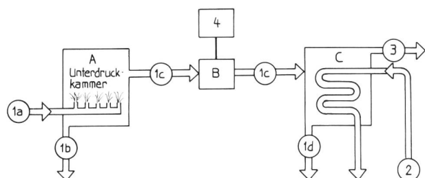
Bild 6. Schema des offenen Kreislaufes – Claude-Zyklus (Zeichnung: Cyrrill Engel ). A Verdampfer, B Niederdruckdampfturbine, C Kondensator, 1 Kreislauf des warmen Oberflächenwassers, 1a Oberflächenwassereintritt, 1b Abfluss von nicht verdampftem Wasser (~ 99,5% von 1a), 1c Niederdruckdampf, 1d entsalztes Wasser, 2 Kühlwasserkreislauf, 3 Gasabzug, 4 Generator.
