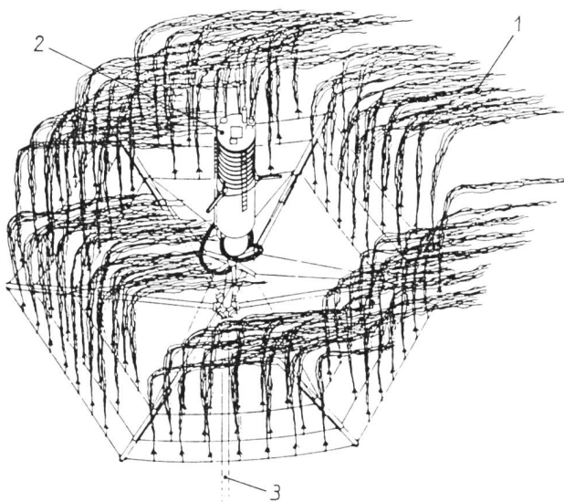
Bild 1. Die Kelpversuchsfarm vor Laguna Beach (Kalifornien). 1 Riesenkelp ( Macrocystis ); 2 Boje mit Instrumenten, Motoren, Pumpe; 3 Nährstoffleitung, 450 m lang, Durchsatz 30000 l/min. Der Aussendurchmesser der Struktur beträgt etwa 32 m (aus: W. J. North, V. A. Gerard, J. S. Kuwabara, W. M. Keck, Caltech: «Biomass Production by Freshwater Marine Macrophytes», 1980).
