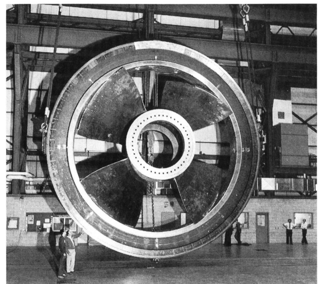
Bild 2. Das Lauftrad der Strafloturbine des Gezeitenkraftwerks Annapolis Royal. Lauftrad mit 7,6 m Durchmesser und 4 festen Schaufeln (Propellerturbine). Gefälle: 1,4 bis 7,1 m; Nennfallhöhe 5,5 m; 378 m 3 Wasser pro Sekunde; 50 U/min; Nennleistung: 17,8 MW. Der fest auf den Schaufeln angebrachte Generator-Rotorring ist deutlich ersichtlich (Foto: Sulzer-Escher Wyss, Zürich).
