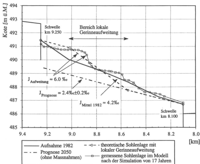
Bild 6. Einfluss der lokalen Gerinneaufweitung auf das Längensprofil.
