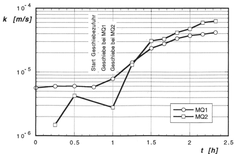
Bild 10. Durchlässigkeitsanstieg beim Feingeschiebetransport.
