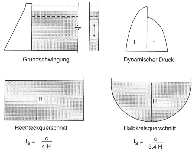
Bild 8. Grundschwingung, dynamischer Druck und Eigenfrequenz bei einfachen Formen des Sees.
