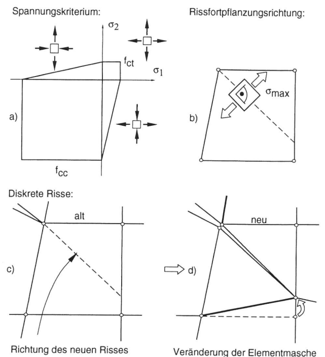
Bild 14. Modell der Rissbildung und -fortpflanzung in Gewichtstaumauern.
