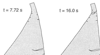
Bild 22. Einfluss einer Verminderung der Zugfestigkeit des Betons von f_{ct} = 2,5 N/mm 2 auf 2 N/mm 2 .
