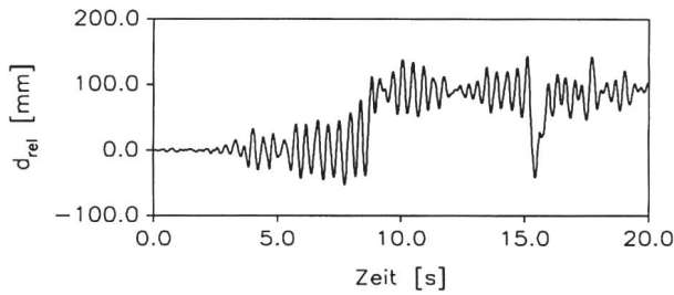
Bild 24. Einfluss einer Veränderung des Zeitverlaufs der Bodenbeschleunigung vom Taft-Beben zum SIA-Beben, beide mit a_{g,max} = 1,8 m/s 2 .
