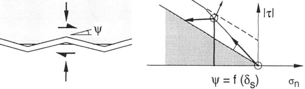
Bild 9. Mechanische Merkmale und zugehörige Stoffgesetze des nichtlinearen Fugenelementes.
