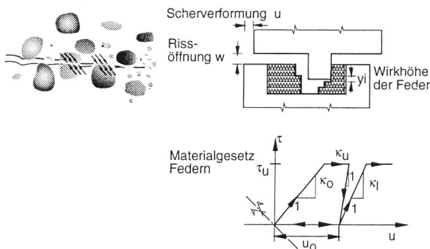
Bild 15. Modell der Risskräfte in Gewichtstaumauern.
