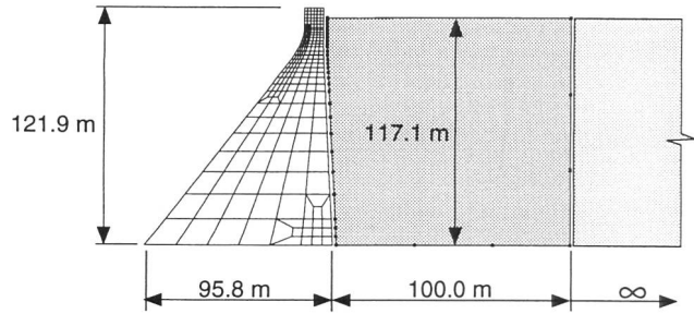
Bild 16. Abmessungen und Modellierung der Pine-Flat-Gewichtstaumauer mit Stausee.
