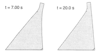
Bild 24. Einfluss einer Veränderung des Zeitverlaufs der Bodenbeschleunigung vom Taft-Beben zum SIA-Beben, beide mit a_{g,max} = 1,8 m/s 2 .
