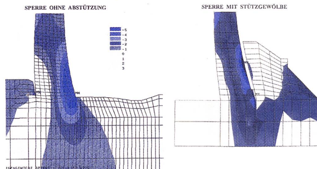
Bild 2. Felsmechanische Untersuchungen für die Sanierung der Kölnbreinsperre. Zonen gleicher Vertikalspannungen bei Vollstau (Schnitt Block 16). Sperre ohne Abstützung (links) und Sperre mit Stützgewölbe (rechts).
