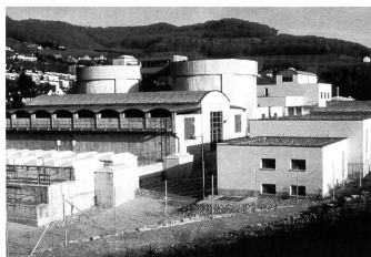
Bild 1. Die neue Kläranlage Ergolz 1 in Sissach.
