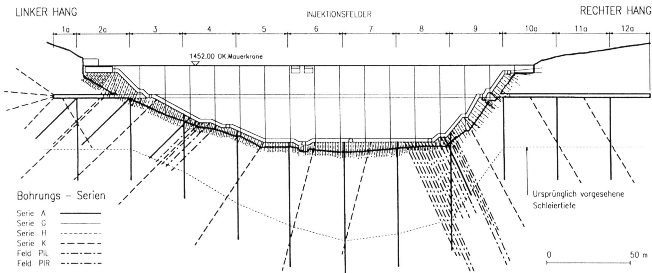
Bild 8. Lage, Verlauf und Tiefe der Bohrungen: Serien A und K (Erkundungs- und Kontrolluntersuchungen); Serien G, H und I (Kontaktinjektionen); linkes und rechtes und Probeinjektionsfelder.
