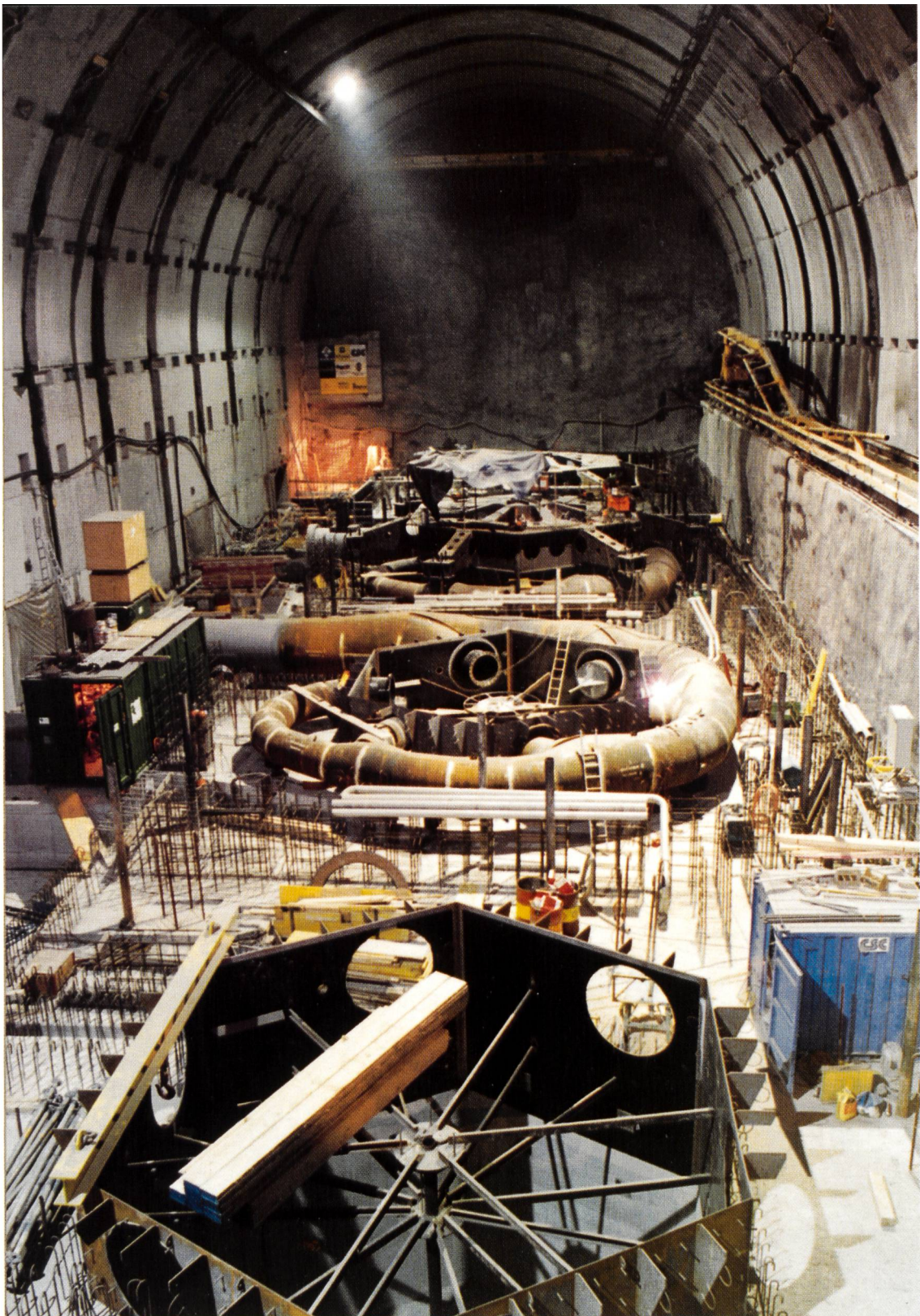
Montage der vier Maschinengruppen in der Kavernenzentrale Amsteg.
