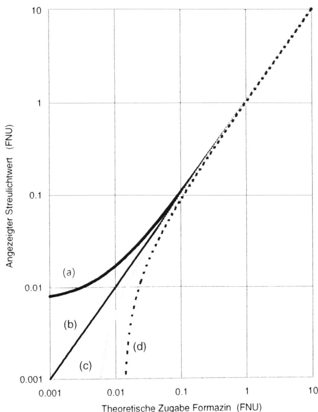
Bild 1. Streulichtanzeige (A) in Funktion der Trübung bei verschiedenen Korrekturen des Nullwerts. Kurve (a): Der Nullpunkt des Geräts ist nicht korrigiert, d. h. der minimale erreichbare Wert entspricht der Grundaufhellung. Kurve (b): Der Nullpunkt ist theoretisch exakt auf den Wert der Grundaufhellung eingestellt. Kurven (c) und (d): Der Nullpunkt ist um 0,03 FNU (c) und 0,05 FNU (d) überkorrigiert; die Anzeige ist zu niedrig und wird bei kleinen Trübungen auch unter Null gehen.
