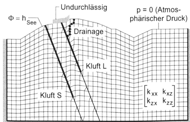
Bild 13. Geometrie, Randbedingungen und Netzeinteilung des Finite-Element-Modelles inkl. der zwei aktiven Klüfte S und L [3].
