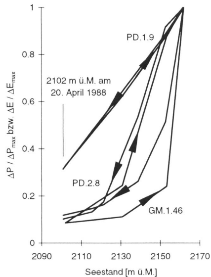
Bild 12. Wechselwirkung zwischen der Kluftöffnung in GM.1 (46 m tief) und dem Wasserdruck an zwei verschiedenen Messstellen in dimensionsloser Darstellung.
