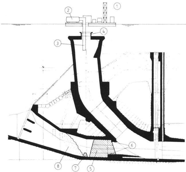
Bild 3. Längensprofil durch den Grundablass einlauf.
