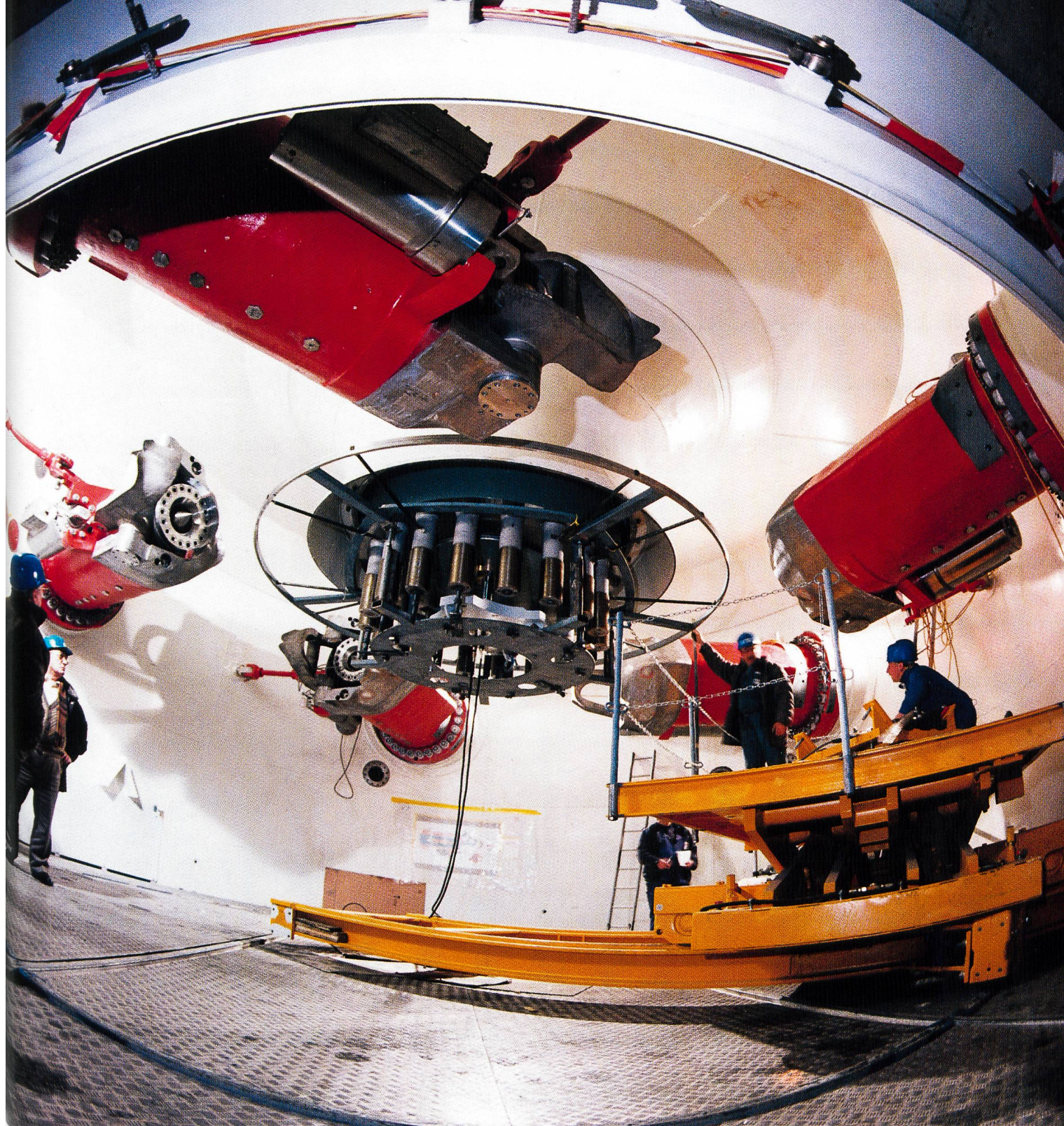
Usine de Bieudron: Derniers réglages avant la pose de la roue Pelton dans le groupe 3 avec une vue sur les injecteurs (Photo: H. Preisig).
