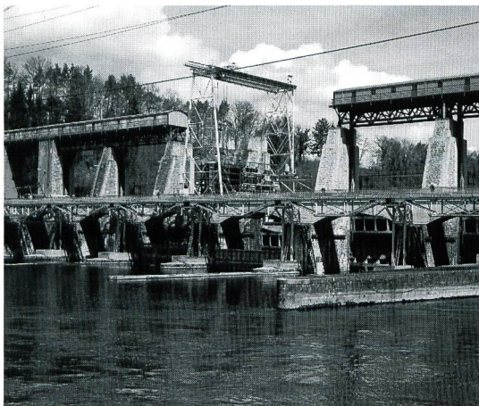
Wasserkraftwerk Eglisau
