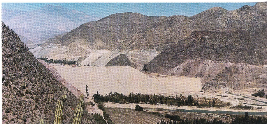
Bild 1. Dammsicht Unterstromseite. Beginn der zweiten Bauphase.
