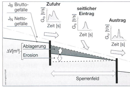
Bild 3. Geschiebebilanzierung innerhalb eines einzelnen Sperrfeldes.
