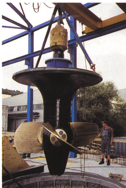
Bild 3. Kernstück, Kaplanlaufrad.
