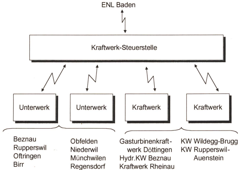
Bild 28. Prinzip der Nachrichtenwege.
