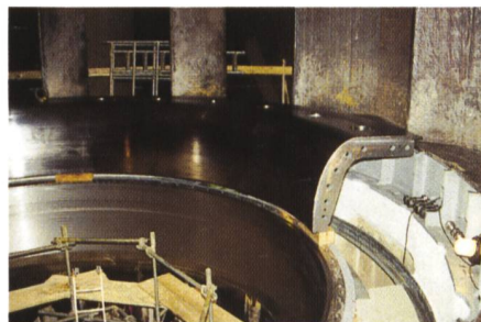
Bild 10. Kraftwerk Wildegg-Brugg: Maschinengruppe 2: Einbau des neuen unteren Leitradringes.
