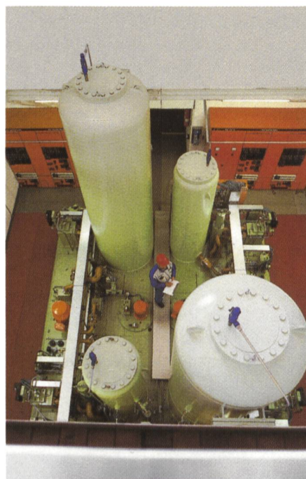
Bild 12. Kraftwerk Wildegg-Brugg: Neue Hydraulikanlagen mit Turbinenregler.
