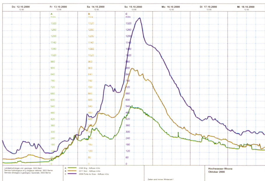
Bild 9. Hochwassersituation an der Rhone 14./15. Oktober 2000: Messwertaufzeichnung [m 3 /s] an den Stationen Brig (unten), Sion (Mitte) und Porte du Scex (oben).
