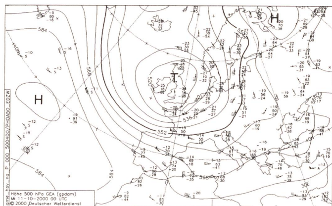
Bild 1. Massgebende Druckverteilung und Strömung (500 mb) am 11. Oktober 2000, 00 UTC (= 2 Uhr mittlereuropäische Sommerzeit MESZ).
