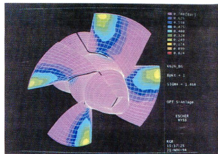
Bild 2. Laufradoptimierung.
