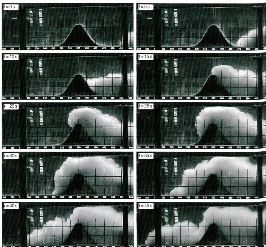
Bild 5. Bildsequenz mit einem Zeitintervall von 5 s eines strömenden Trübestroms, der von rechts nach links über ein Hindernis fliesst (Versuch B01).
