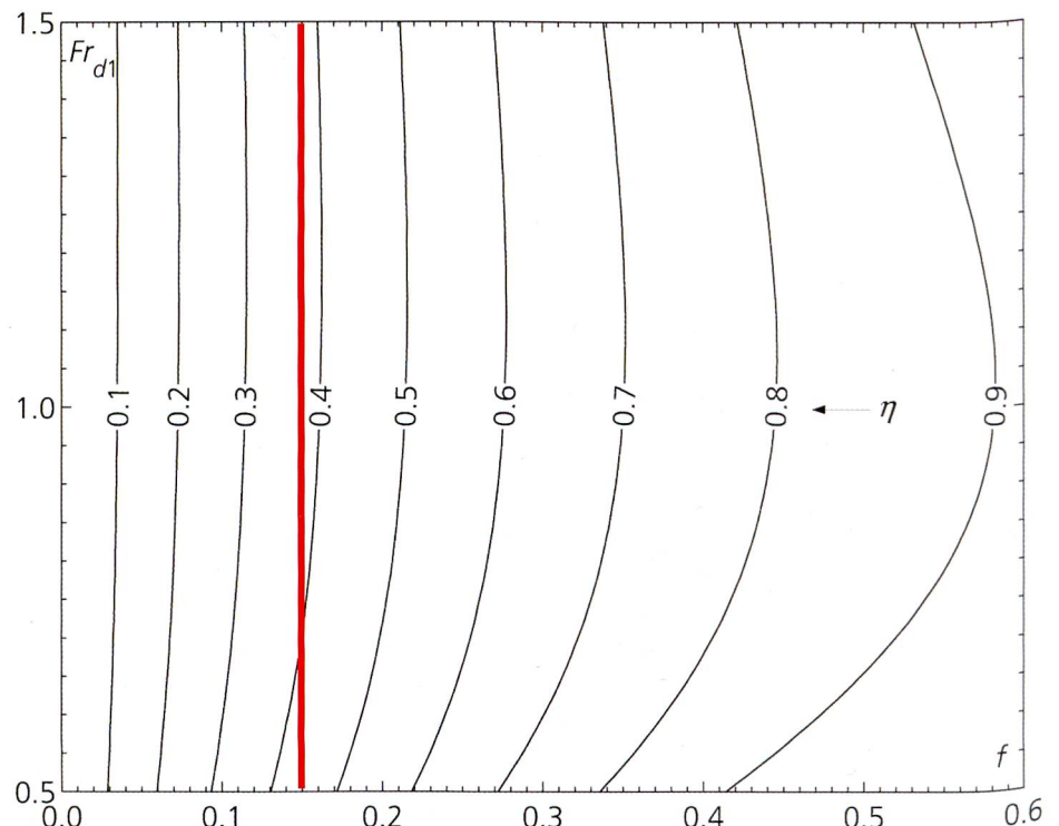
Bild 10. Sedimentdurchgängigkeit \eta eines Gitters in Abhängigkeit der wirksamen Porosität f und der Froudezahl des ankommenden Trübestromes Fr_{dt} .
