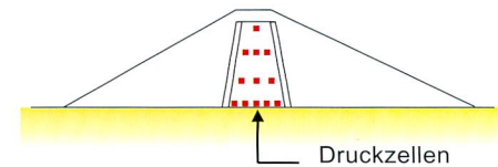
Bild 9. Schüttdamm mit zentralem Kern. Verteilung der Druckmesszellen.
