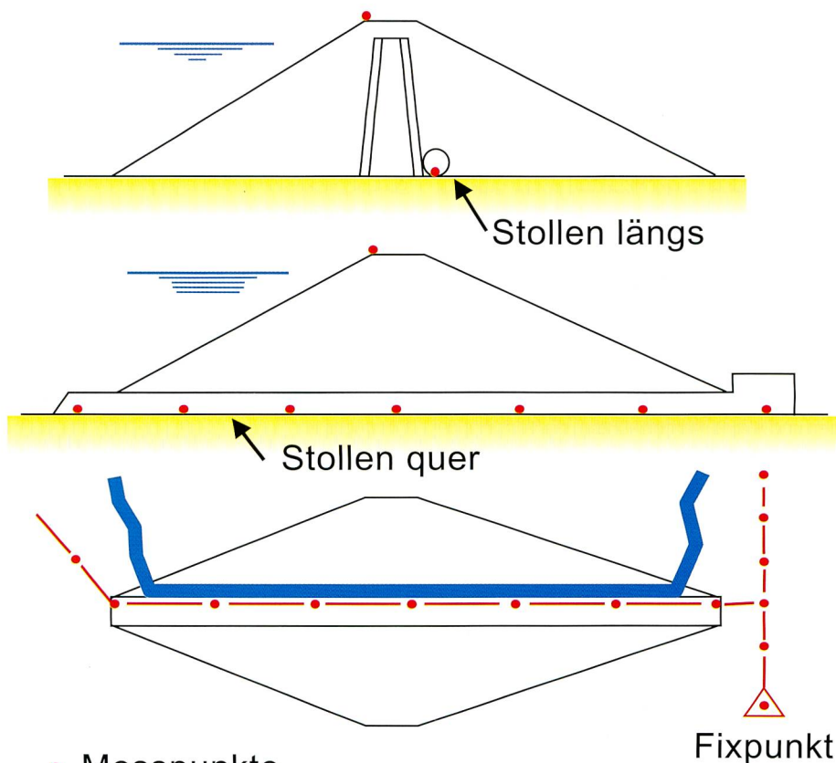
Bild 4. Damm. Messung der Deformationen auf Höhe der Dammkrone und in einem Stollen.
