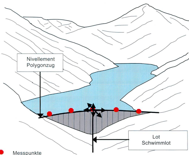
Bild 2. Staumauer. Messung der Deformationen auf der Höhe der Kronenkote.
