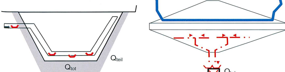
Bild 7. Staumauer und Damm. Sickerwassermessungen Q_{total} und Q_{teil} .
