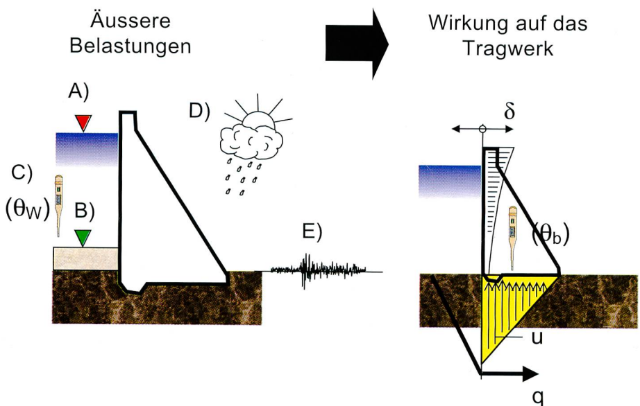
Bild 1. Wirkungen der äusseren Belastungen auf das Bauwerk. Äussere Belastungen: A) Wasserdruck; B) Druck aus Sedimenten; C) Wassertemperatur; D) klimatische Verhältnisse (Lufttemperatur, Regen, Schnee); E) Belastung durch Erdbeben. Wirkungen der Lasten: Verformungen ( \delta ); Betontemperaturen ( \theta_b ); Durchsickerungen ( q ); Auftrieb ( u ) und Porenwasserdrücke.
