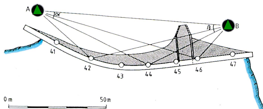
Bild 4. Damm. Messung der Deformationen auf Höhe der Dammkrone und in einem Stollen.
