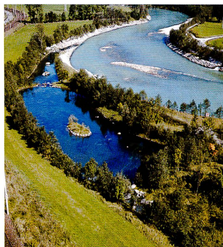
Bild 4. Umgehungsbach als Fischauftiegshilfe, Kraftwerk St. Veit an der Salzach.
