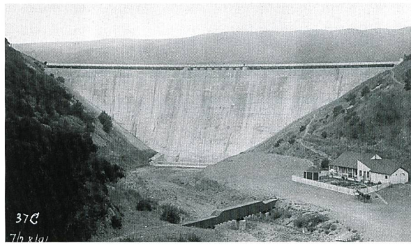
Bild 5. Die Lower-Crystal-Springs-Gewichtsmauer in unmittelbarer Nähe der San-Andreas-Verfugung hat die starken Erschütterungen des San-Francisco-Erdbebens von 1906 schadlos überstanden. Die 44,5 m hohe Mauer besteht aus verzahnten Betonblöcken, und bei starker seismischer Beanspruchung können sich kurzfristig einige der Fugen öffnen. Als 1887 mit dem Bau dieser Mauer begonnen wurde, war dies weltweit die grösste Staumauer. Die Mauer wurde 1911 erhöht (Foto: City of San Francisco).
