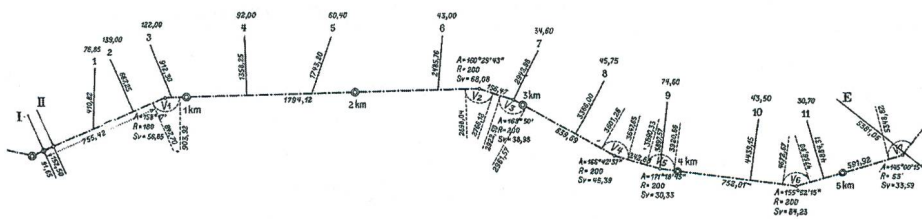
Abb. 10. Schematischer Lageplan des Zulaufstollens. Legende: I Schacht am See, II zweiter Schacht, 1 bis 11 Seitenstollen bzw. „Fenster“, E Ende des Zulaufstollens beim Wasserschloss.
