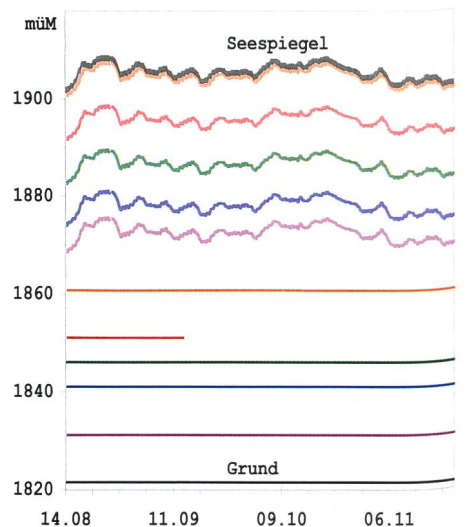
Bild 7. Knoten des Seespiegels und der Temperatursensoren vor der Bogenmauer im Herbst 2000. Zum Vergleich liegt der Abfluss des Sees durch den Gelmerstollen auf 1833 m ü.M., die Fassung des Werks Grimsel 2 im Bereich des Chessiturms auf 1842 m ü.M.
