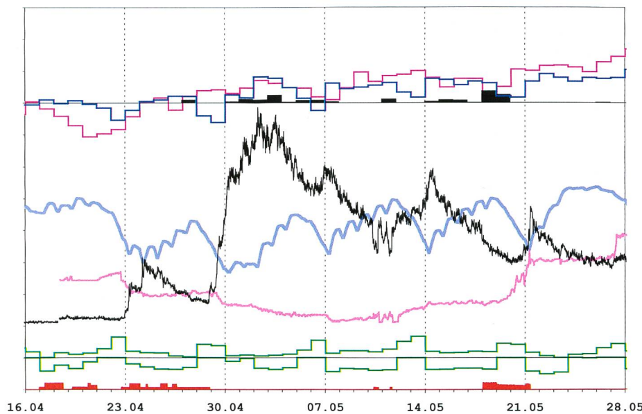
Bild 6. Ausschnitt aus Bild 5. Das Absetzen von Eismassen im Grimselsee auf Grund, erkennbar an reduzierten oder «negativen» Seezuflässen (dunkelblaue Treppenlinie oben) bei sinkendem Seespiegel (blau), löste nach dem Wochenende vom 21./22. April 2001 und an den vier folgenden Wochenenden jeweils einen Anstieg der Trübung im Tiefenwasser aus (schwarz).
