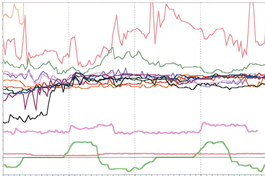
Bild 9. Temperaturverlauf vor der Spittelamm Sperre ab Dienstag, 24. August 2000, mittags (Skala von 4,5 bis 6,5 °C). Sondenpositionen siehe Legende Bild 10. Auf der Horizontalachse unten sind Trübesignal (mit Offset) und Abflüsse im Grimsel 2 sowie Abflüsse aus dem See aufgetragen (Skalen siehe Bild 10).
