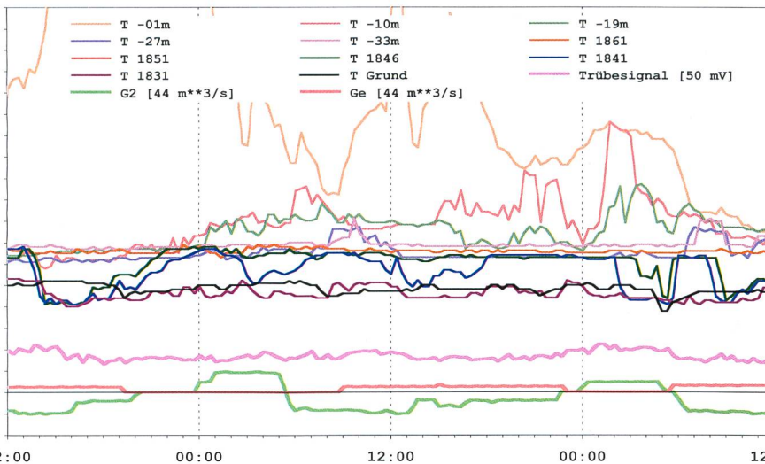
Bild 10. Temperaturverlauf über die Seetiefe vor der Spittelamm Sperre ab Mittwoch, 4. Oktober 2000, mittags (Skala von 5 bis 7 °C) sowie Trübesignal (mit Offset) und Abflüsse im Gelmerstollen (Ge) und Abflüsse im Grimsel 2 (G2). Die Skaleneinheit, d.h. der Abstand zwischen benachbarten Skalenstrichen, ist in eckiger Klammer angegeben.
