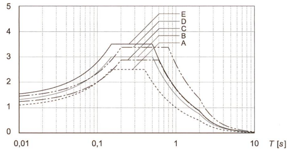
Bild 2. Elastische Beschleunigungsantwortspektren der SIA-Norm 261 (2003) für 5%-Dämpfung für verschiedene Baugrundklassen (A = Fels) und einer Spitzenbodenbeschleunigung von a_{gd} (Wiederkehrperiode: 475 Jahre).
