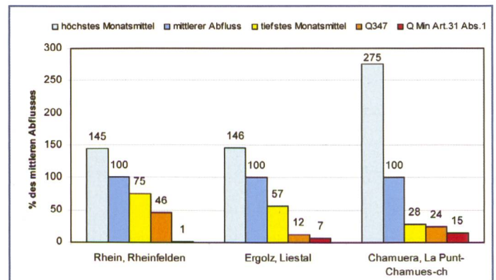
Bild 4. Unterschiedliche Abflusswerte verschiedener Fließgewässer aus dem Alpenraum und Mittelland (mittlerer Abfluss = 100%). Datenquelle: www.bafu.admin.ch/hydrologie .
