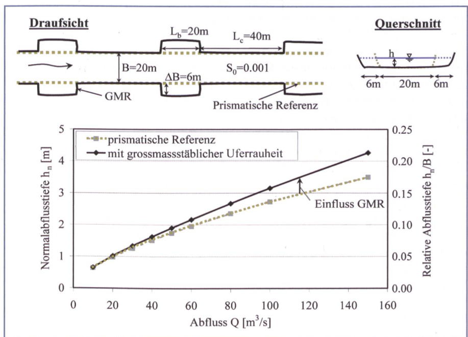
Bild 8. Berechnungsbeispiel für die Normalabflusstiefe unter Berücksichtigung von grossmassstäblichen Uferauheiten.
